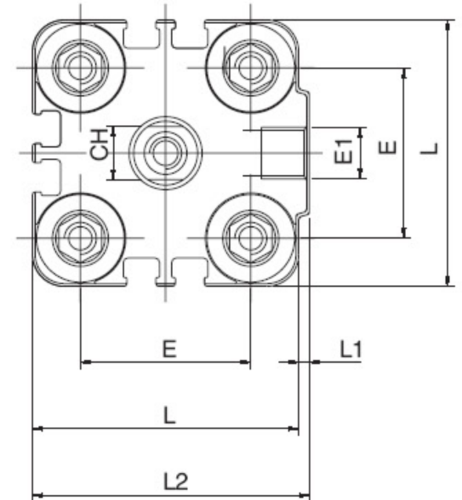
D32-40-50-63-80-100
